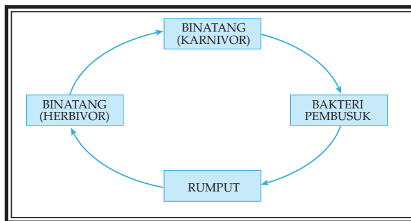
Gambar 4.1 Skema rantai makanan dalam satu lingkungan. (Sumber: diolah oleh Gnaya, 2006)
