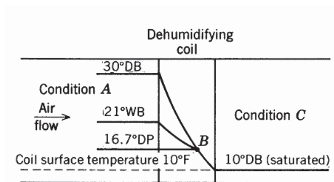
Gambar 4.11 Sketsa Proses Pendinginan dan pengurangan uap air
