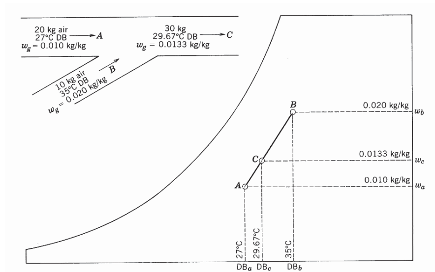
Gambar 4.13 Ilustrasi Pencampuran Udara
