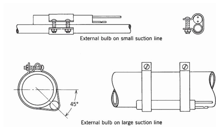
Gambar 9.8 Detail contoh pemasangan remote bulb
