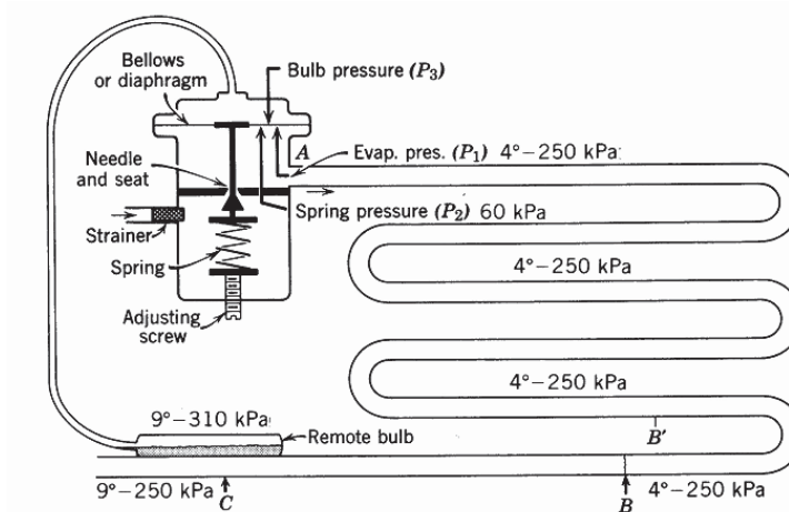
Gambar 9.9 Ilustrasi prinsip kerja katub ekspansi thermostatik
