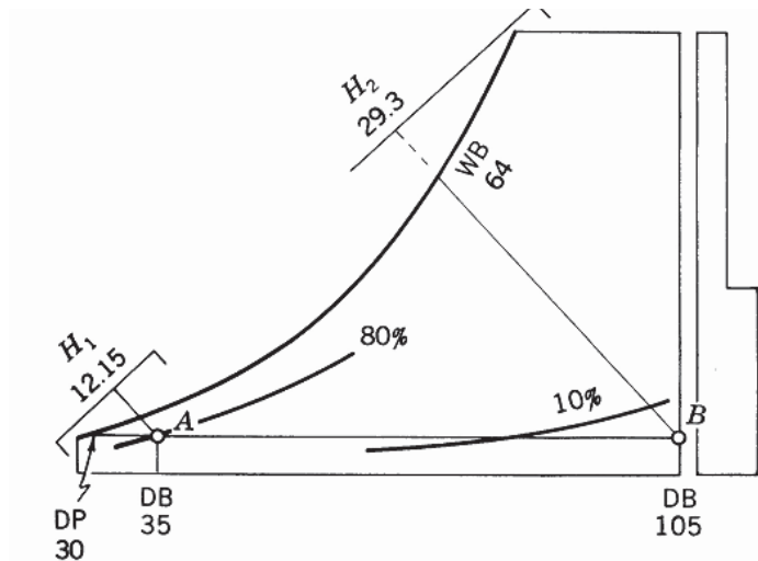
Gambar 4.7 Hasil Pemetaan pada Psikrometrik Chart Contoh 4.2
