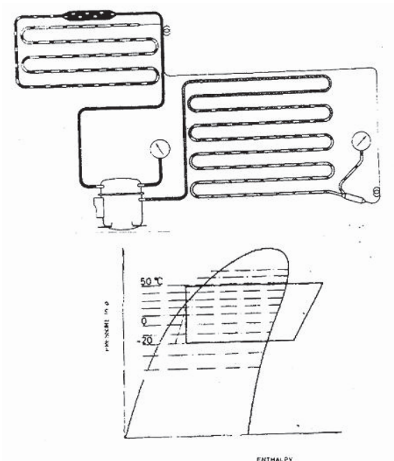
Gambar 5.9. Siklus Refrigeran
