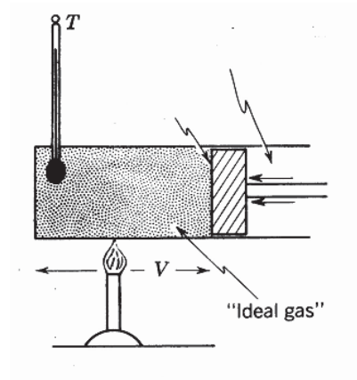
Gambar 3.2 Gas di dalam silinder dipampatkan sedemikian sehingga suhu gas tetap konstan.
