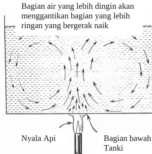
Gambar 2.2 Konduksi
