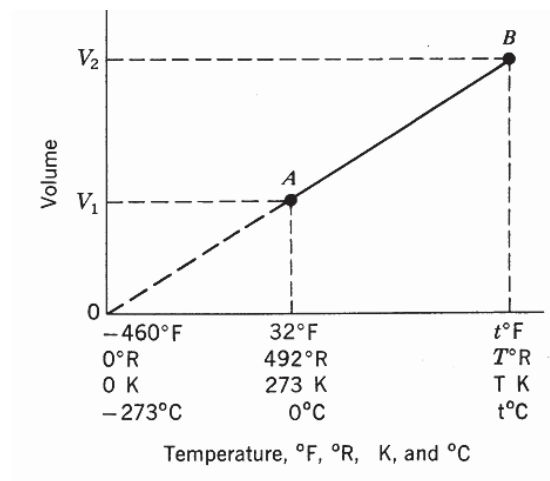
Gambar 3.3 Kurva V-T. Dari kurva V-T yang merupakan garis lurus diketahui bahwa ratio dua variabel pada titik A dan titik B mempunyai nilai sama, sehingga (V_1)/(V_2) = (T_1)/(T_2) .
