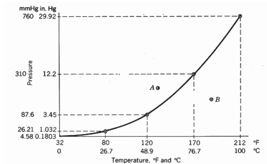
Gambar 2.17 Kurva P-T atau Kurva Titik Didih Air
