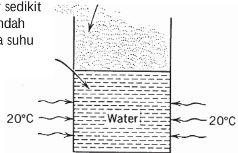
Gambar 3.8 Evaporasi dari permukaan air yang ada di dalam bejana terbuka.
