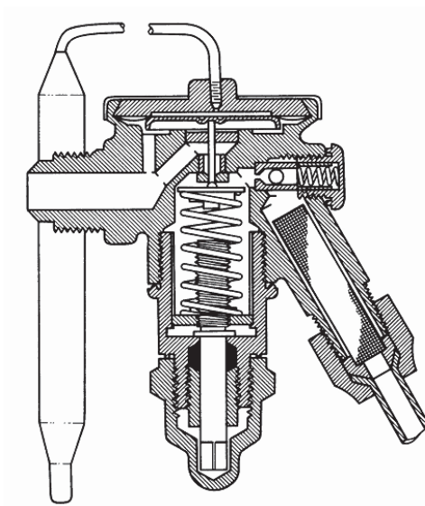
Gambar 9.6 Ilustrasi konstruksi katub ekspansi thermostatik
