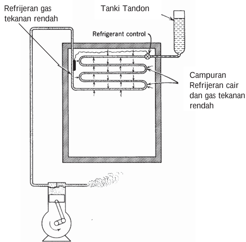
Gambar 5.5 Tipikal koil evaporator yang dilengkapi dengan katub ekspansi thermal atau thermostatic expansion valve
