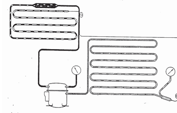
Gambar 5.12 Efek Kondensasi di Kondenser
