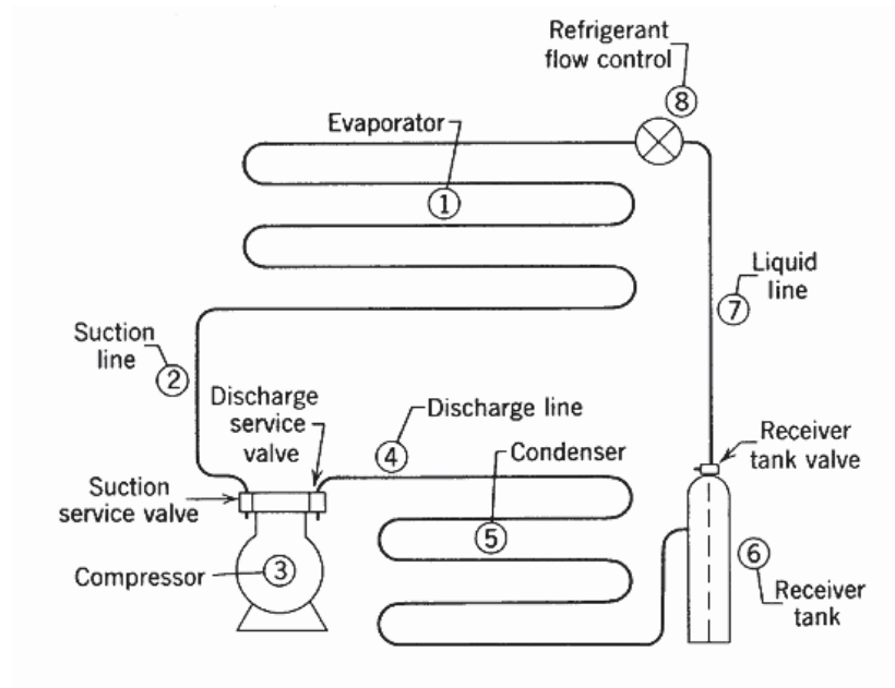
Gambar 5.7 Diagram Alir sistem Kompresi Gas
