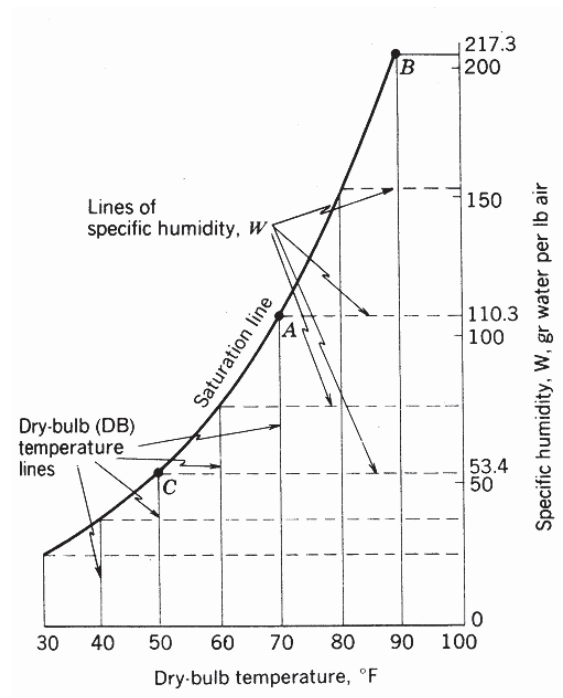
Gambar 4.2 Tipikal pemetaan garis skala Suhu bola kering (DB), Kelembaban Spesifik (specific humidity, w ), dan garis saturasi (saturation line)
