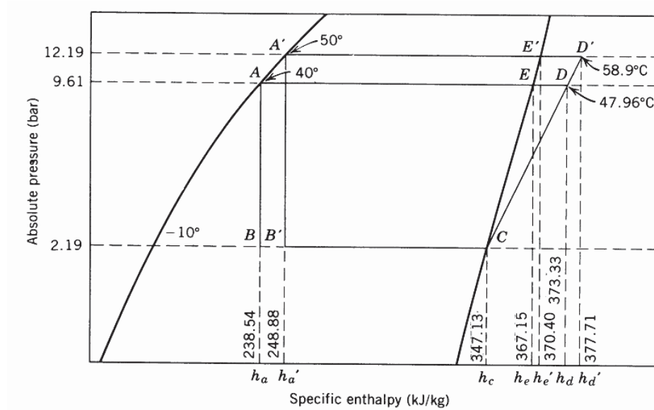
Gambar 6.7 Pemetaan dua Suhu Kondensasi yang berbeda
