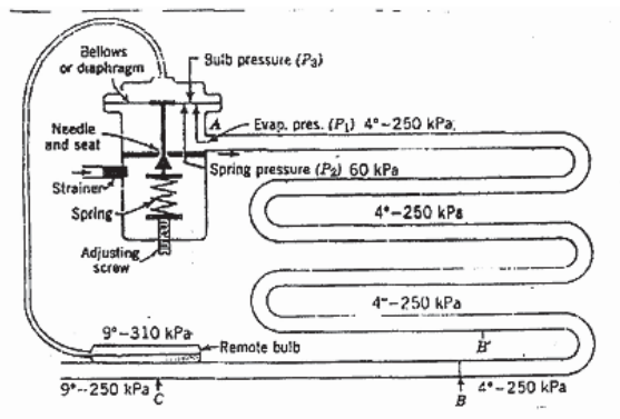
Gambar 5.13. Efek Ekspansi di Katub Ekspansi
