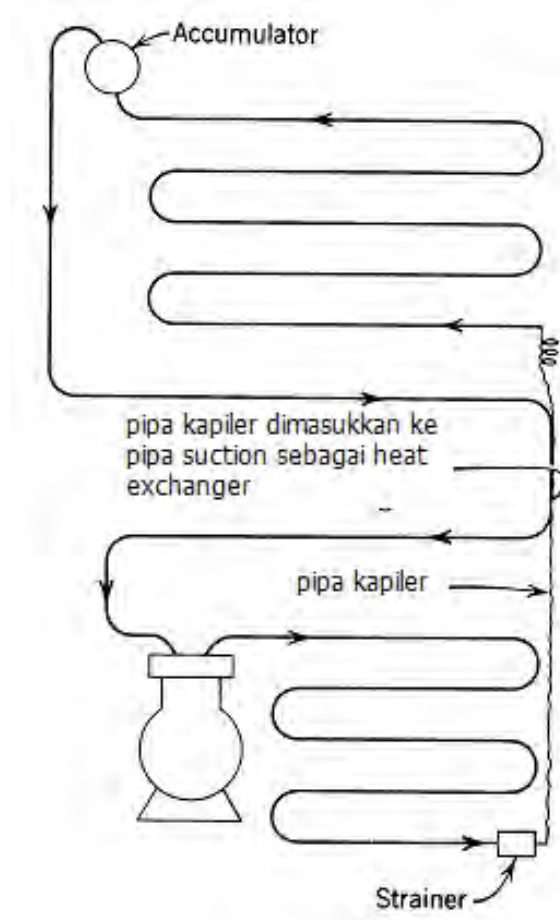
Gambar 9.13 Sistem Pipa Kapiler
