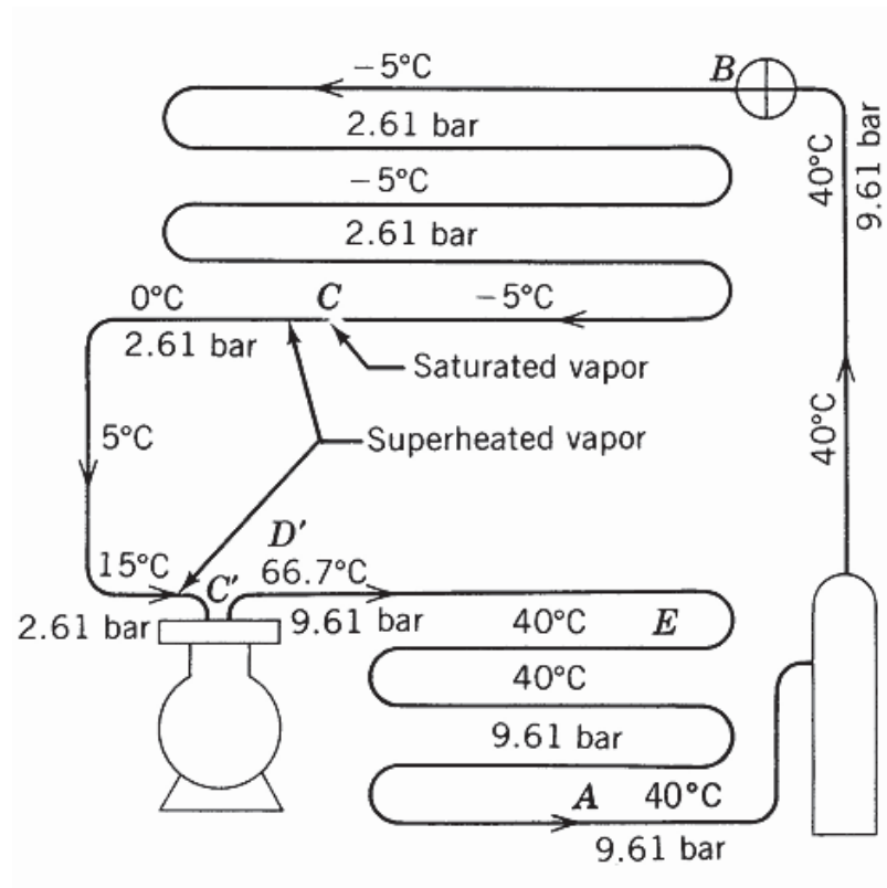
Gambar 5.14 Tipikal actual Proses
