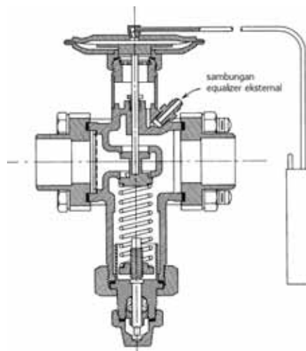
Gambar 9.12 Konstruksi katub ekspansi dengan equalizer eksternal
