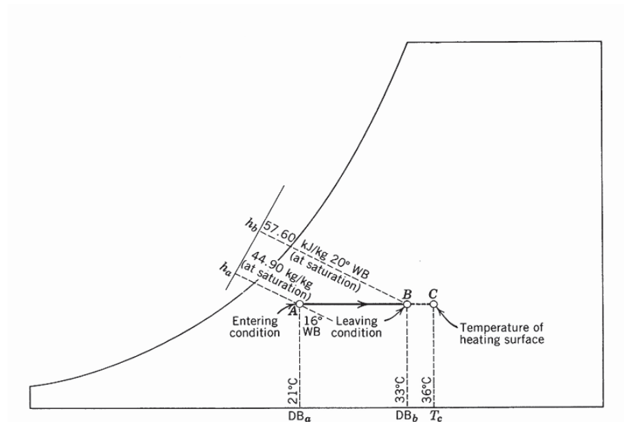
Gambar 4.8 Pemetaan Proses Pemanasan Sensibel
