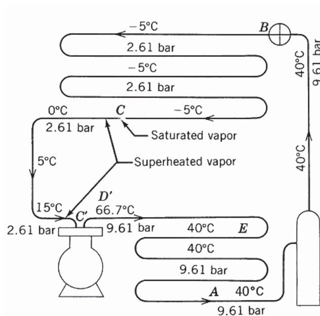
Gambar 6.8 Diagram aliran untuk proses gas panaslanjutan.
