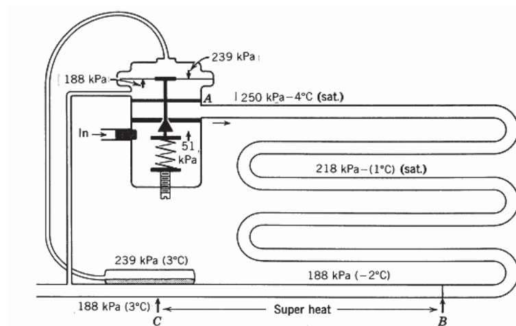
Gambar 9.12 Konstruksi katub ekspansi dengan equalizer eksternal
