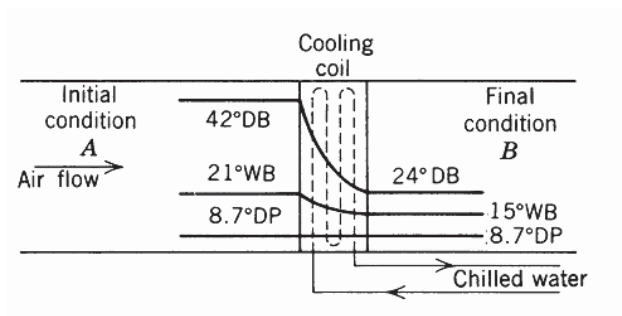
Gambar 4.10 Pemetaan proses pendinginan sensibel
