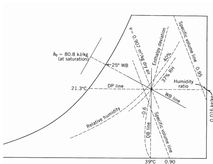
Gambar 4.1 Tipikal pemetaan garis skala Psikrometrik chart
