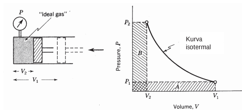
Gambar 3.1 Gas di dalam silinder dikompresi tetapi suhu gas dipertahankan konstan. Dari kurva P-V diketahui, bahwa area yang ada di bawah kurva memiliki luas sama, yaitu (P_1)(V_1) = (P_2)(V_2) .
