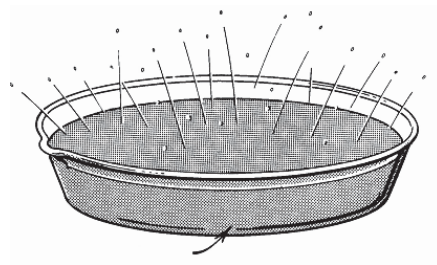
Gambar 3.7 Evaporasi yang berlangsung pada permukaan liquid
