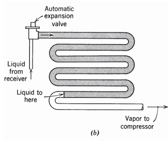
Gambar 9.5 Kondisi refrijeran pada saat beban evaporator minimum
