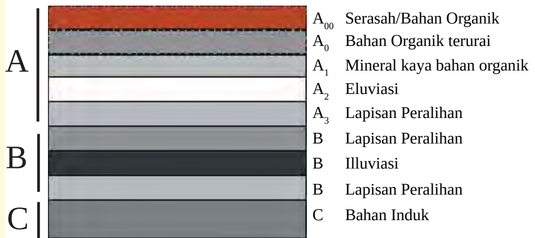
Gambar 8.32 Profil Tanah
