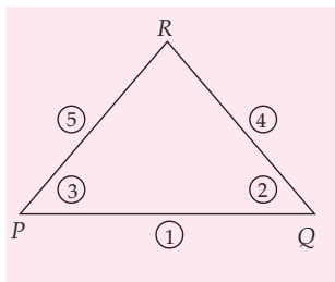
Gambar 8.52 Segitiga PQR
