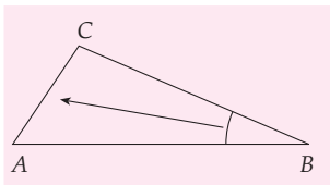
Gambar 8.37 Segitiga ABC
