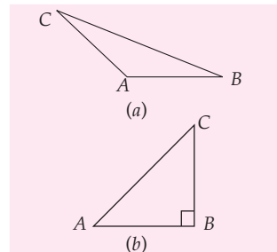
Gambar 8.40 (a) Segitiga tumpul, (b) Segitiga siku-siku
