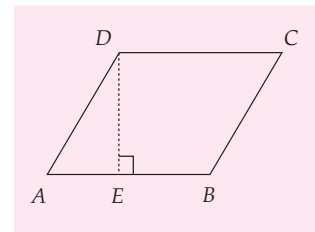
Gambar 8.28 Jajargenjang ABCD
