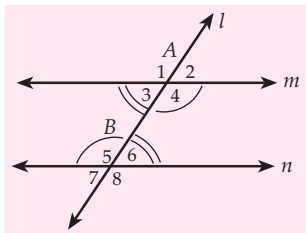
Gambar 7.35 Pasangan sudut dalam berseberangan.
