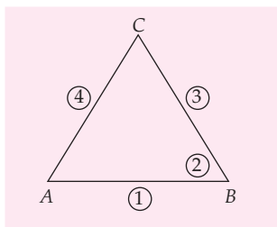
Gambar 8.53 Segitiga ABC
