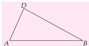
Gambar 8.9 Segitiga ABD
