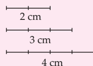
Gambar 8.50 Segitiga dengan sisi 2 cm, 3 cm, dan 4 cm
