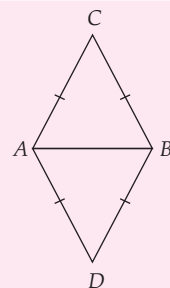
Gambar 8.16 Sisi-sisi belah ketupat sama panjang
