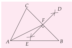
Gambar 8.45 Melukis garis sumbu
