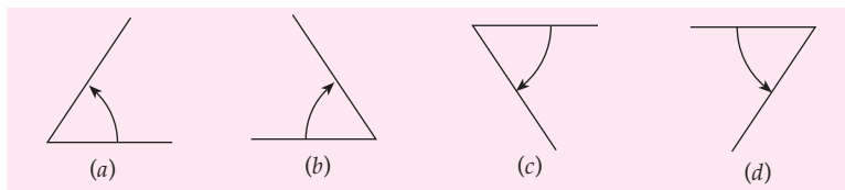
Gambar 7.18 Sudut lancip.
