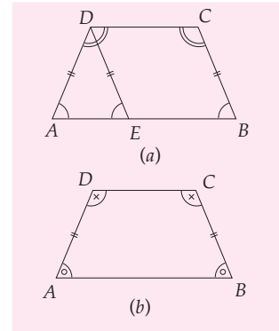
Gambar 8.25 (a) Trapesium ABCD sama kaki, (b) trapesium ABCD sama kaki dengan \angle A = \angle B dan \angle C = \angle D
