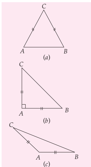
Gambar 8.41 (a) Segitiga lancip sama kaki; (b) Segitiga siku-siku sama kaki; (c) Segitiga tumpul sama kaki
