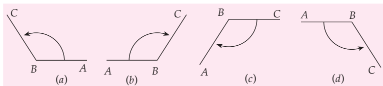
Gambar 7.20 Sudut tumpul.
