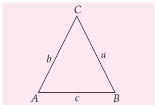
Gambar 8.59 Segitiga ABC
