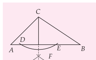
Gambar 8.42 Melukis garis tinggi
