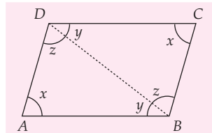
Gambar 8.12 Jajargenjang ABCD dengan sudut-sudut yang berhadapan sama besar
