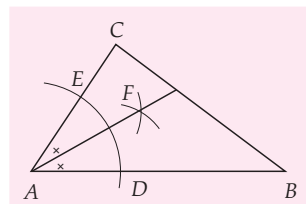
Gambar 8.43 Melukis garis bagi
