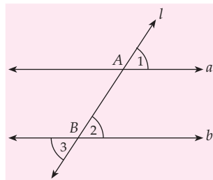
Gambar 7.46 Garis a \parallel b jika sudut-sudut luar berseberangan sama
