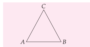
Gambar 8.39 Segitiga lancip
