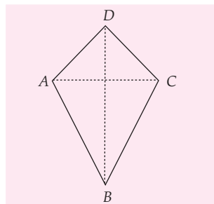
Gambar 8.22 Diagonal BD merupakan sumbu simetri pada layang-layang
