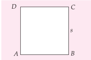
Gambar 8.31 Persegi ABCD
