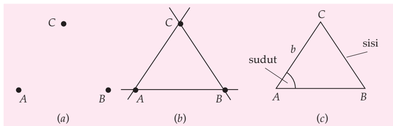
Gambar 8.36 Unsur-unsur segitiga
