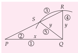
Gambar 8.54 Segitiga PQS dan segitiga PQR
