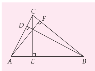
Gambar 8.60 Segitiga ABC
