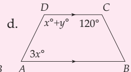
Gambar 8.26 Trapesium ABCD sama kaki dengan AC = BD
