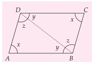
Gambar 8.14 Jumlah sudut-sudut yang berdekatan adalah 180^\circ
