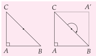
Gambar 8.5 Persegi ABA'C
