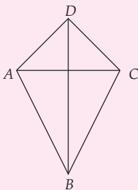
Gambar 8.33 Layang-layang ABCD
