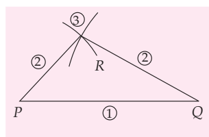
Gambar 8.51 Segitiga PQR
