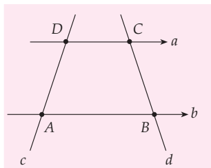
Gambar 8.6 Trapesium ABCD
