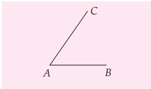
Gambar 7.8 Sudut BAC
