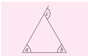
Gambar 8.58 Jumlah a dan b adalah c
