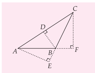
Gambar 8.61 Segitiga ABC
