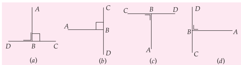
Gambar 7.19 Sudut siku-siku.
