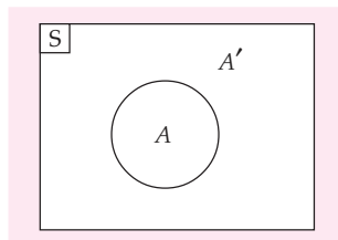
Gambar 6.10 Komplemen A
