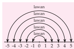
Gambar 1.4 Garis bilangan
