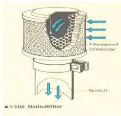
Gambar 5.5: saringan udara
