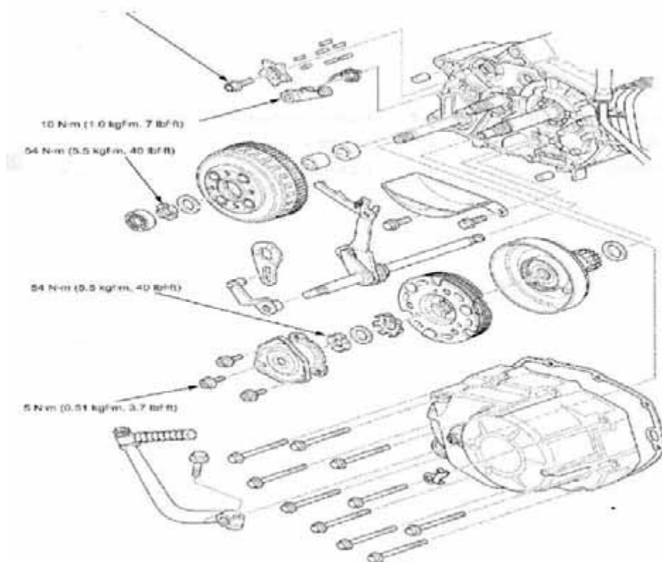
Gambar 6.16: melepas unit kopling dari mesin
