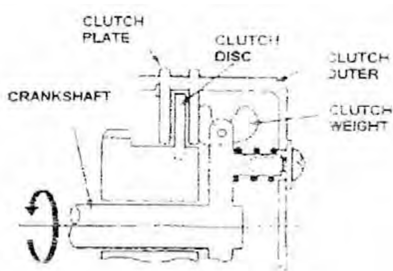
Gambar 6.5: kopling otomatis posisi terlepas
