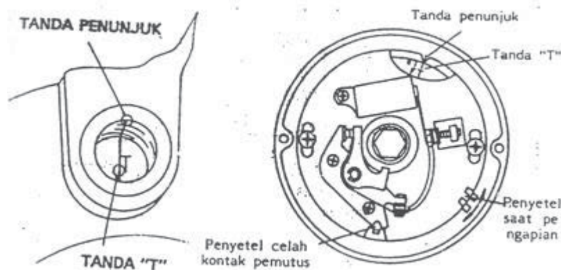
Gambar 1.11: tanda "penunjuk" pada poros engkol
