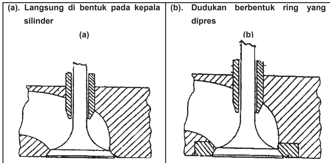
Gambar 1.6: macam macam dudukan katup (a&b)
