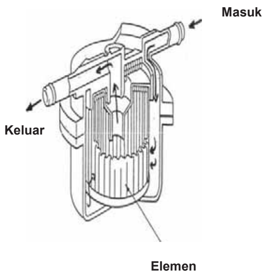
Gambar 5.4: saringan bensin
