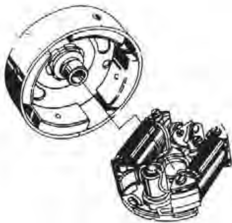
Gambar 2.6 generator pembangkit
