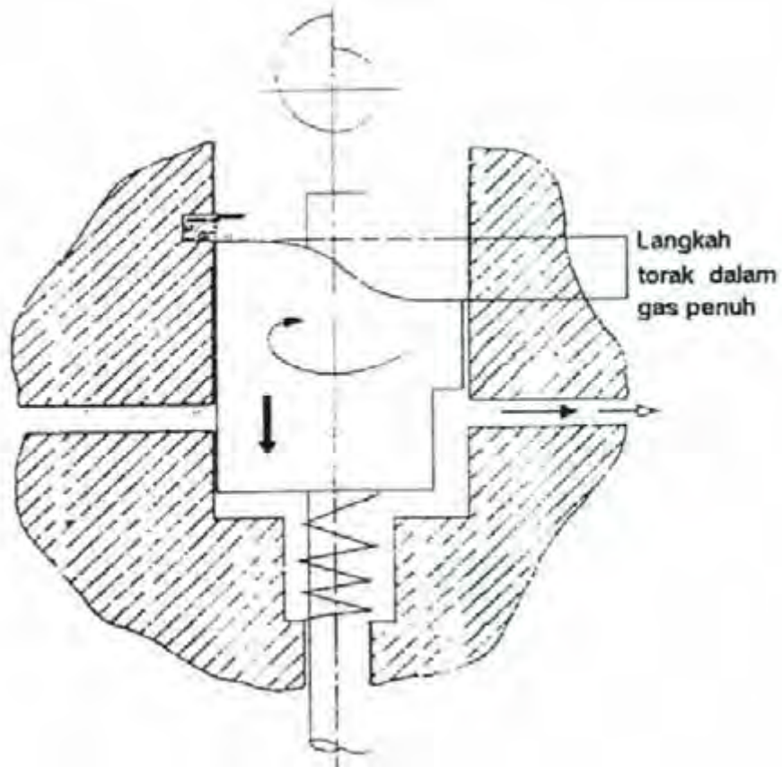
Gambar 3.12: posisi gas penuh (akhir langkah tekan)
