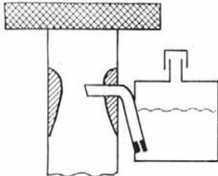
Gambar 5.9: ventilasi ekstern
