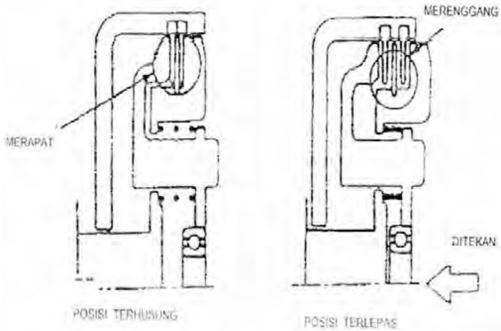
Gambar 6.3: kopling posisi terhubung (kiri) dan posisi terlepas (kanan)
