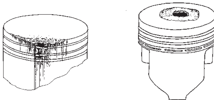
Gambar 2.56: piston rusak/cacat
