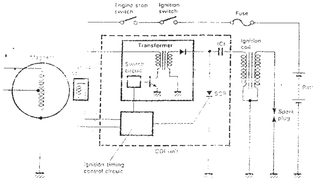
Gambar 2.40: rangkaian sistem pengapian CDI - DC
