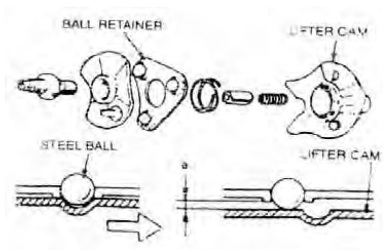
Gambar 6.7: proses pemindahan gigi
