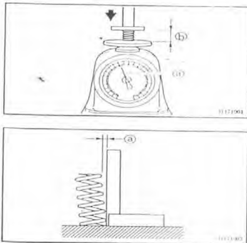
Gambar 6.22: pemeriksaan pegas kopling
