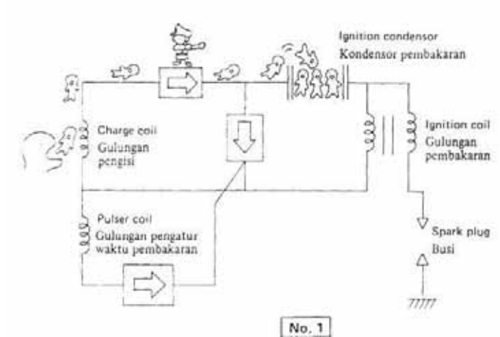
Gambar 2.37: tegangan disearahkan oleh diode
