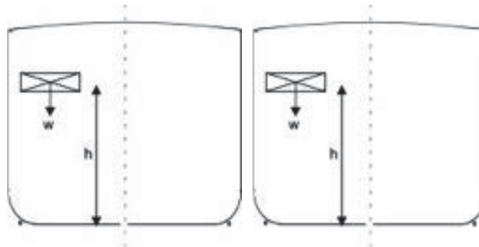
Gambar 6.3 Momen komponen kapal terhadap keel
