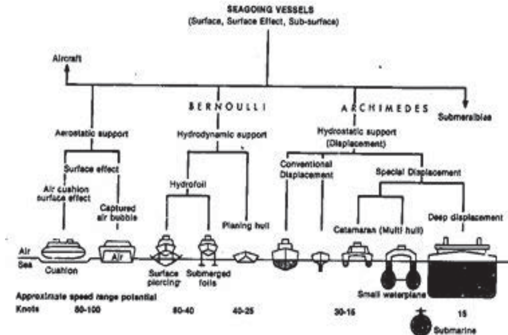
Gambar 2.22 Diagram pohon pengelompokan kapal menurut garis air.
