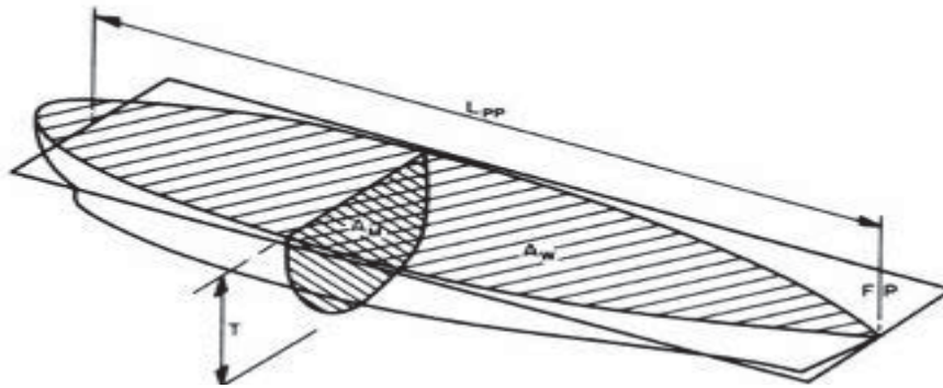
Gambar 5.5 Koefisien Blok
