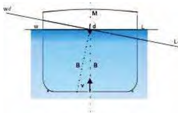
Gambar 6.12 Momen Inersia melintang.
