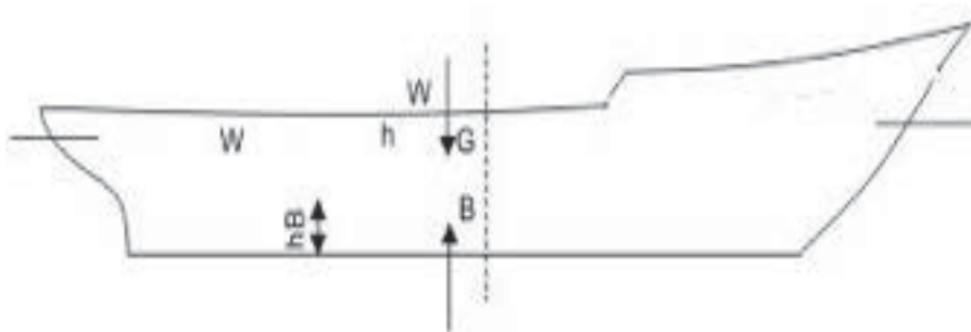
Gambar 6.6 Garis vertical dari titik tekan dan titik berat
