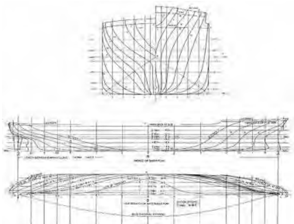
Gambar 5.1 Rencana garis air/Half breadth/Waterlines plan menunjukkan interseksi
