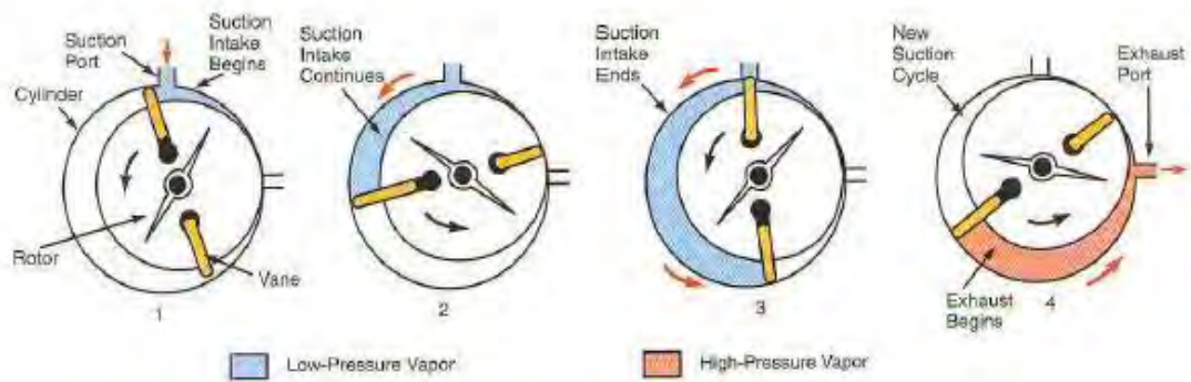
Gambar 2. 17 Kompresor Rotari
