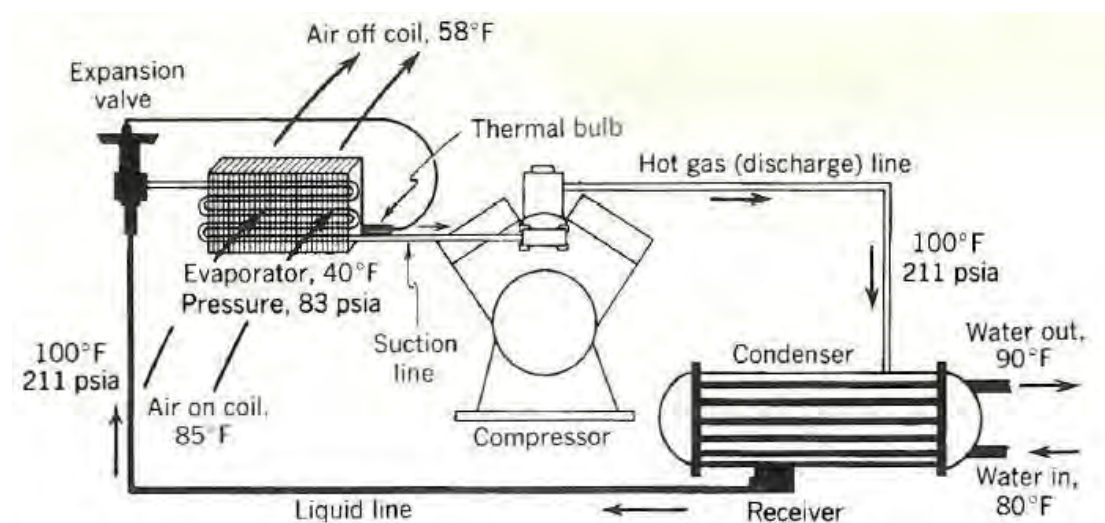
Gambar 2. 1 Tipikal Sistem Refrigerasi Kompresi Gas
