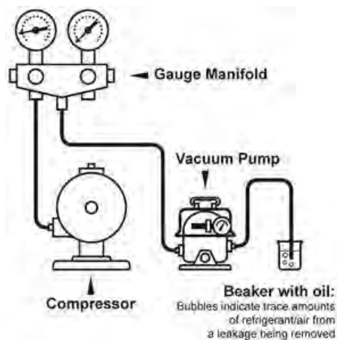
Gambar 4. 18 Pengujian Kebocoran
