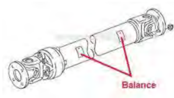
Gambar 4.54. Pemeriksaan keseimbangan/balance poros propeler
