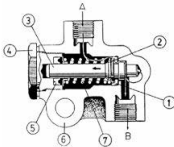
Gambar 2.89.Kontruksi Katup Proporsional
