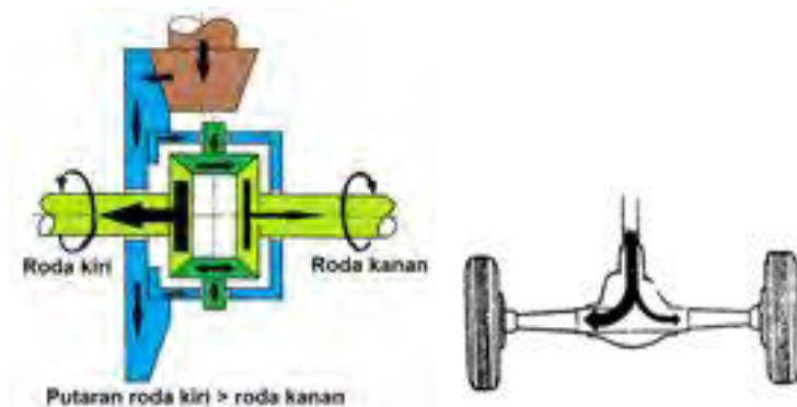
Gambar 4.66. Cara kerja diferensial saat belok
