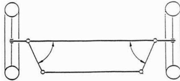
Gambar 3.17. Kemudi lengan trapesium posisi lurus
