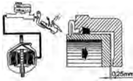
Gambar 2.26. Sil Torak kaliper lepas injakan
