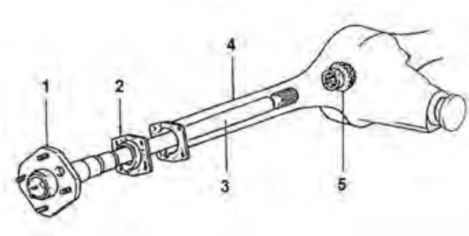
Gambar 4.40. Konstruksi poros roda pada aksel rigid
