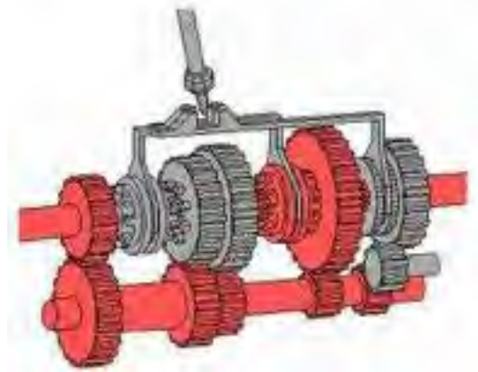
Gambar 4.28. Transmisi tanpa sinkromesh
