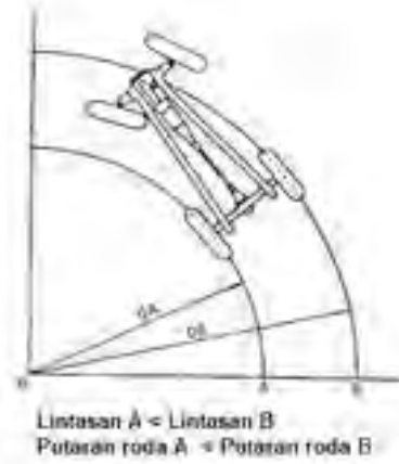
Gambar 4.63. Fungsi diferensial
