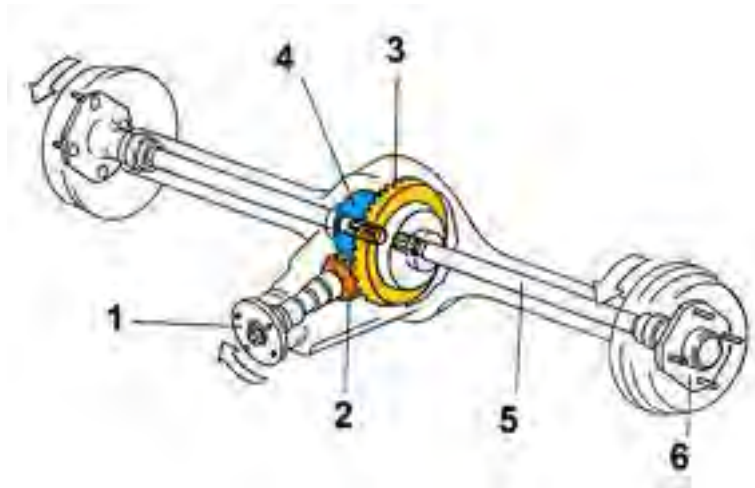
Gambar 4.55. Penggerak Aksel
