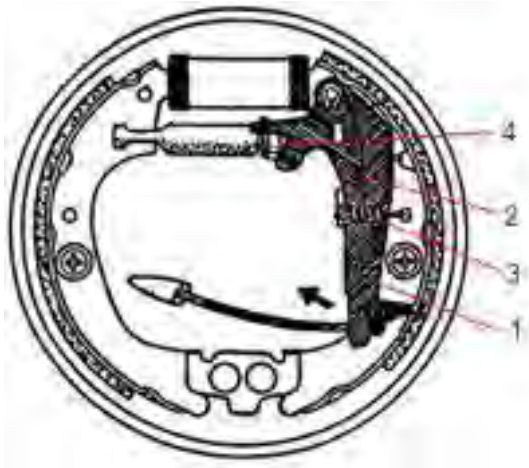
Gambar 2.73.Konstruksi Penyetelan Otomatis Rem Tangan Pada Rem Tromol
