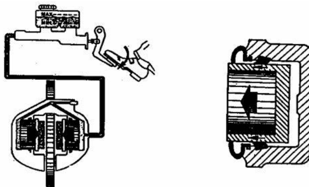
Gambar 2.25. Sil Torak kaliper bertekanan
