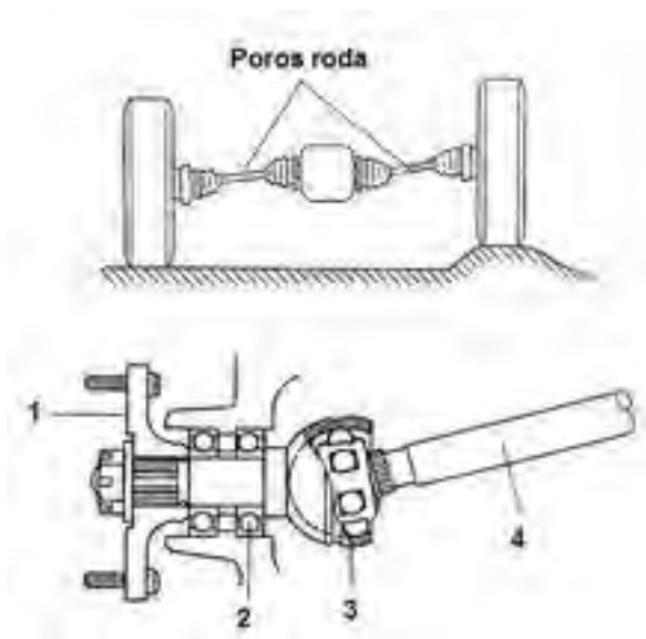
Gambar 4.41. Konstruksi Poros roda pada Aksel Independen
