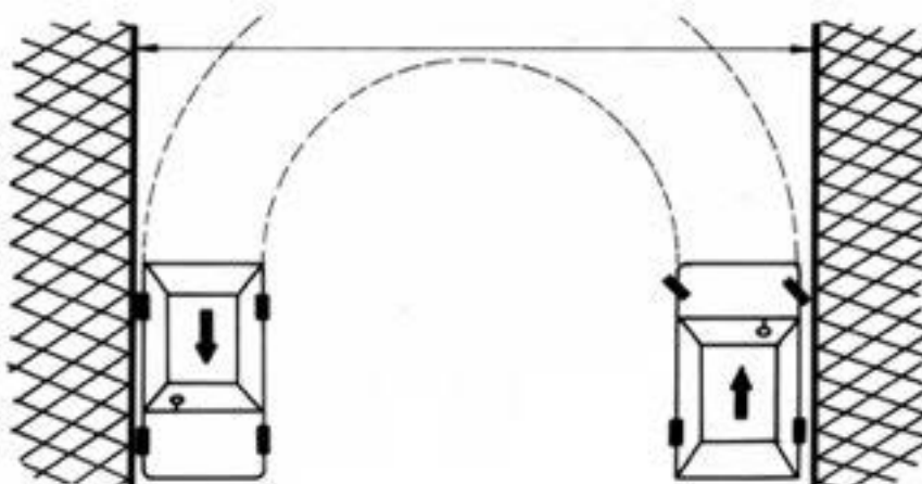
Gambar 6.9. Sudutputarmaksimum kendaraan
