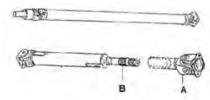
Gambar 4.39. Fungsi bagian-bagian poros penggerak aksel
