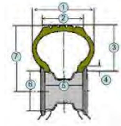
Gambar 7.13. Ukuran Ban
