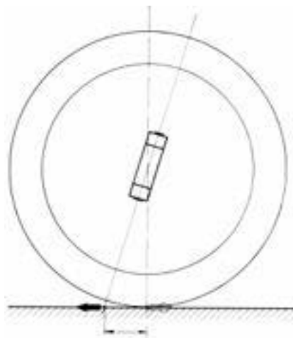
Gambar 6.12. Caster
