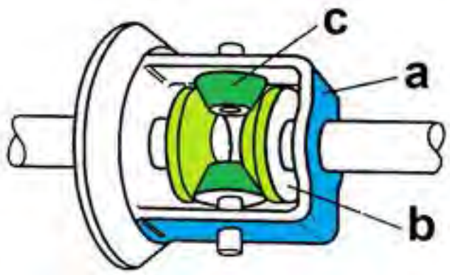
Gambar 4.64. Bagian-bagian diferensial
