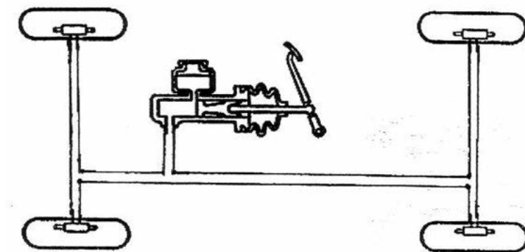
Gambar 2.32.Hidraulik rem satu sirkit
