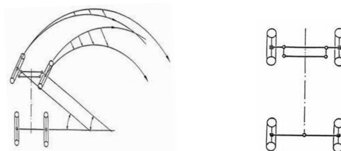
Gambar 3.15. Kemudi lengan paralel
