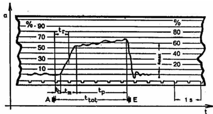
Gambar 8.4 Grafik Hasil Pengukuran Perlambatan
