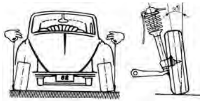
Gambar 6.16. Camber negatif
