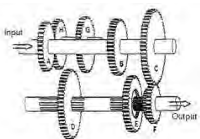
Gambar 4.26. Transmisi dua poros
