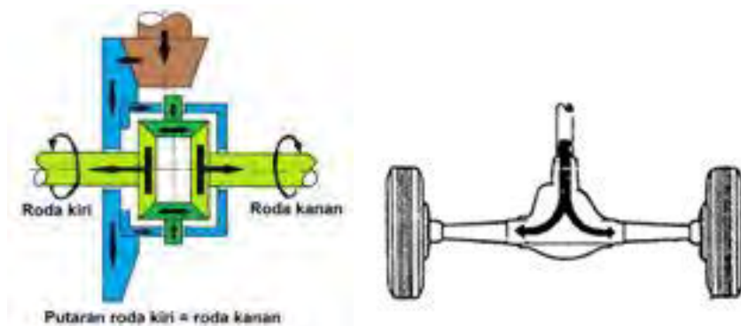
Gambar 4.65. Cara kerja diferensial saat lurus
