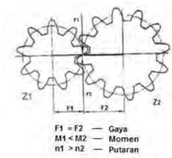
Gambar 4.23. Konsep pemindahan putaran dan momen pada roda gigi
