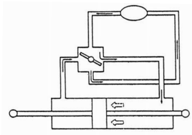
Gambar 3.25. Prinsip kerja hidrolik power steering saat belok
