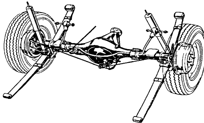
Gambar 5.47. Contoh pemasangan stabilisator (3)
