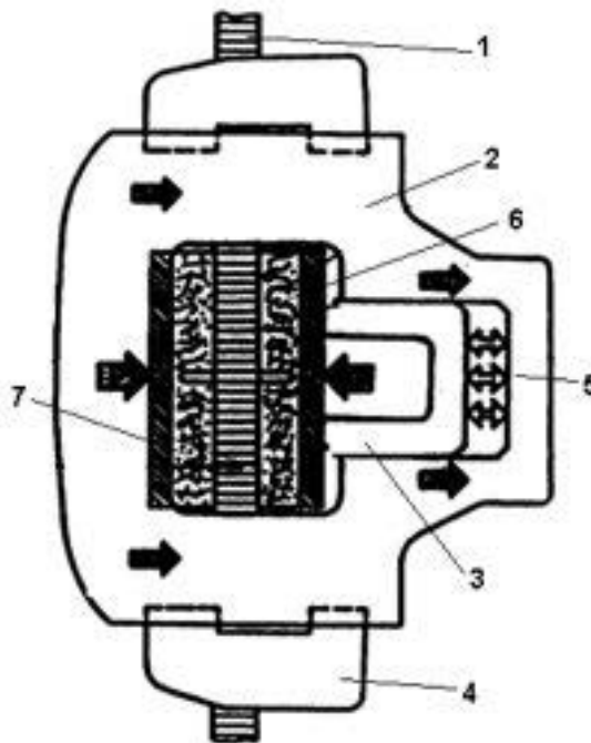
Gambar 2.21. Kaliper Luncur satu Torak
