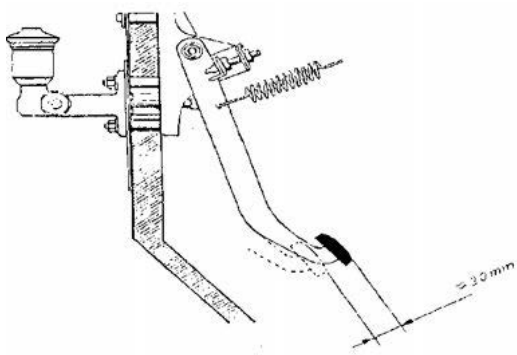
Gambar 4.18. Pemeriksaan kebebasan pedal kopling
