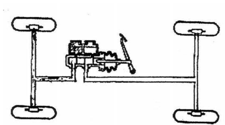
Gambar 2.33.Hidraulik rem dua sirkuit aksial
