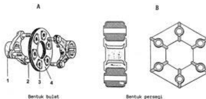
Gambar 4.44. Penghubung fleksibel
