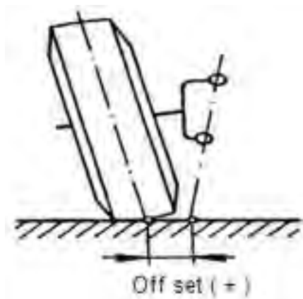
Offset positif
