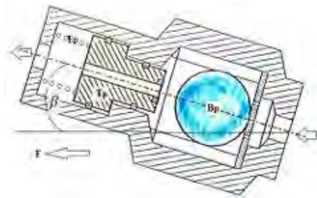
Gambar 2.95. Kontruksi Katup Pengatur Bola Perlambatan
