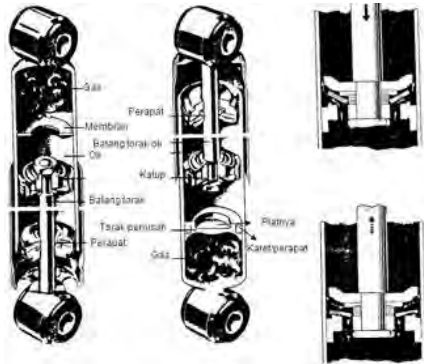
Gambar 5.52. Peredam getaran satu pipa
