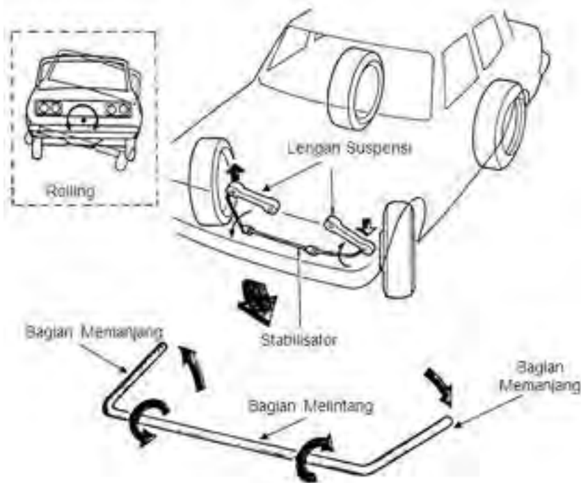
Gambar 5.44. Stabilisator
