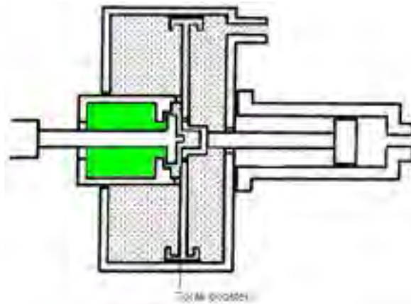
Gambar 2.64. Prinsip Kerja Boster Saat Lepas Injakan
