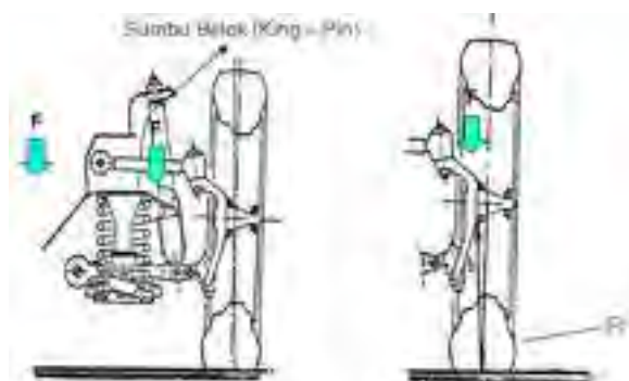
Gambar 6.18. Letak beban spindel camber positif
