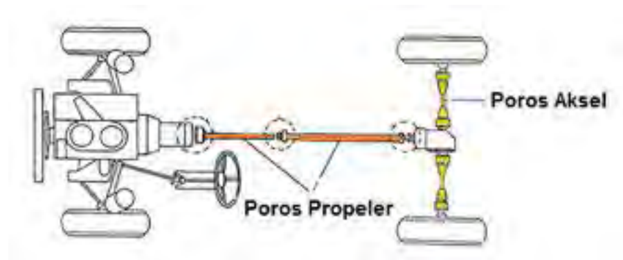
Gambar 4.37. Posisi poros penggerak dalam sistem pemindah tenaga
