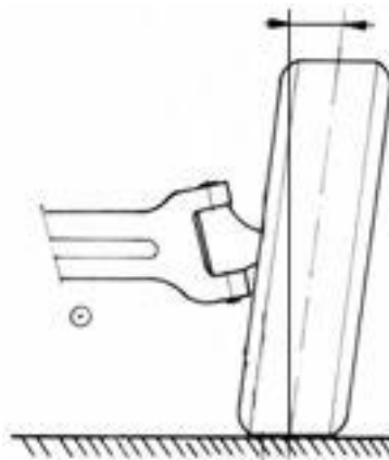
Gambar 6.11. Camber
