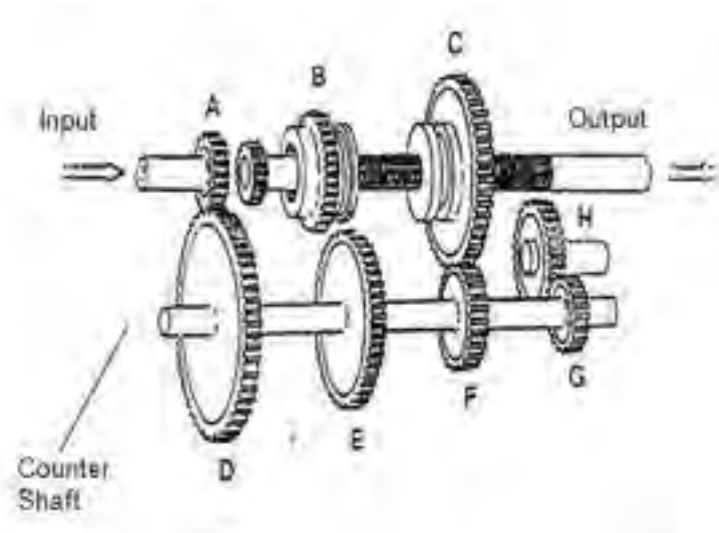
Gambar 4.27. Transmisi tiga poros
