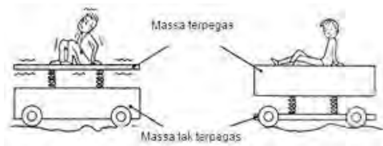
Gambar 5.39. Prinsip pemegasan
