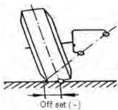
Gambar 6.38. Offset nol, negatif dan positif
