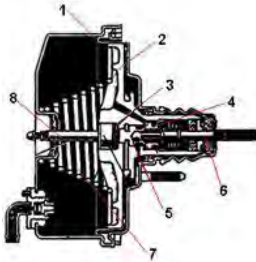
Gambar 2.61.Konstruksi Boster
