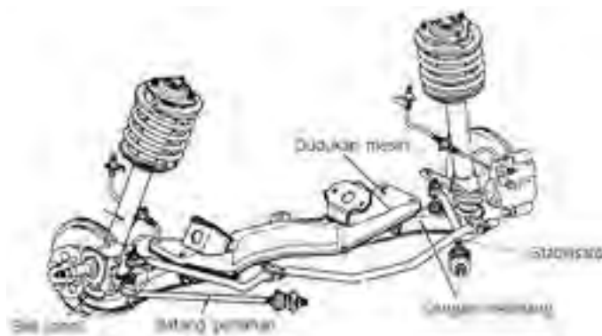
Gambar 5.30. Mac. Pherson Lengan melintang dan batang penahan
