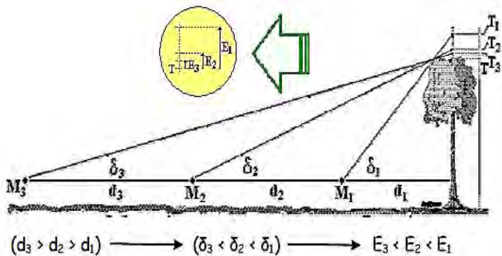
Gambar 67. Ilustrasi upaya memperkecil kesalahan ukur tinggi bertajuk lebar
