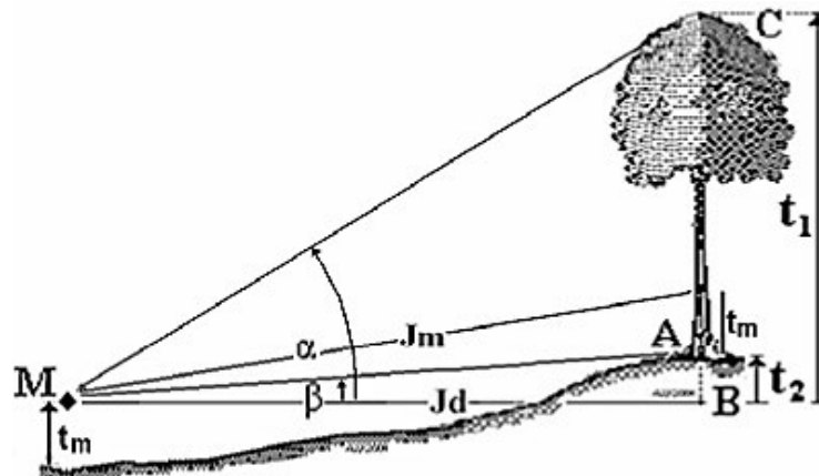
Gambar 28. Rumus dasar tinggi berdasarkan posisi (3)
