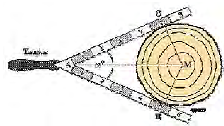
Gambar 38. Cara penggunaan garpu pohon
