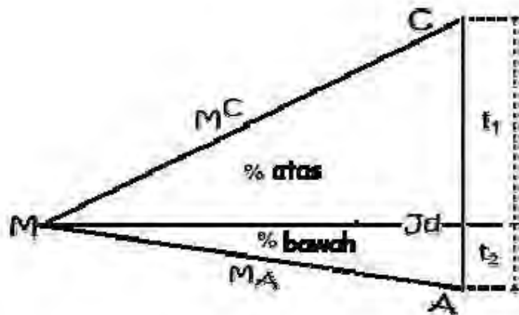
Gambar 31. Dasar pembacaan persen sudut
