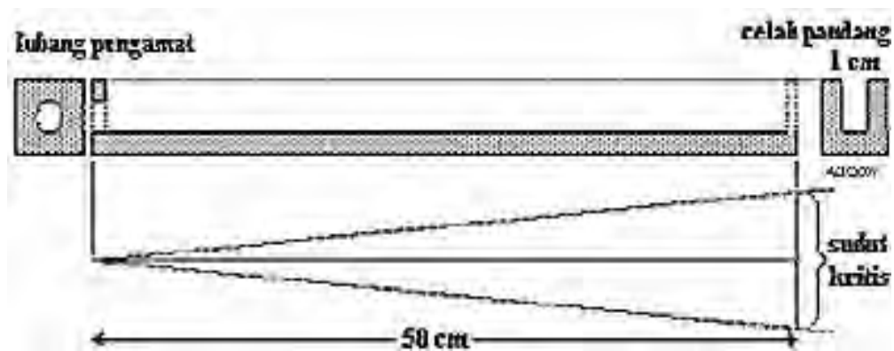
Gambar 44. Tongkat Bitterlich dengan nilai K = \frac{1}{50} .
