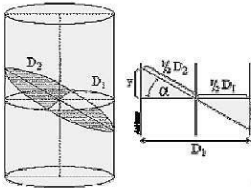
Gambar 37. Kesalahan ukur pada penggunaan kaliper
