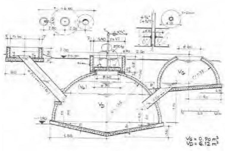
Gambar 20. Konstruksi reaktor biogas (Jerman)
