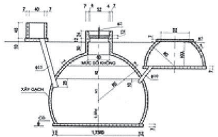
Gambar 21. Konstruksi reaktor biogas (Vietnam)
