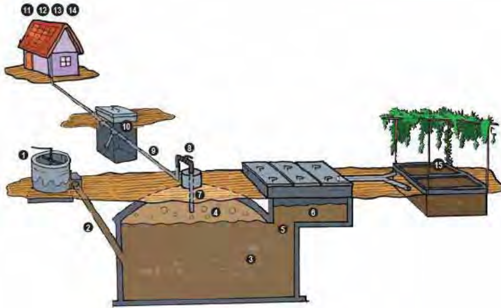
Gambar 39. Komponen reaktor biogas
