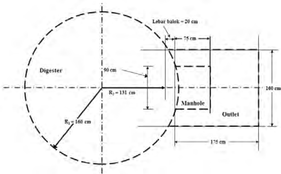
Gambar 181. Dimensi reaktor biogas ukuran 6\text{m}^3
