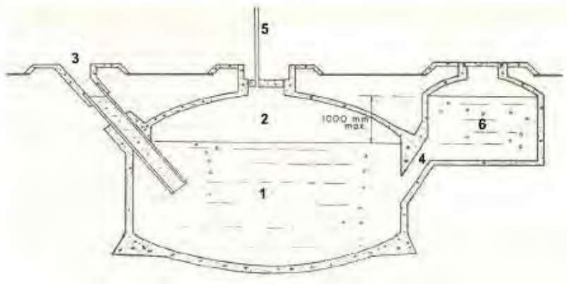
Gambar 23. Konstruksi reaktor biogas (Cina)
