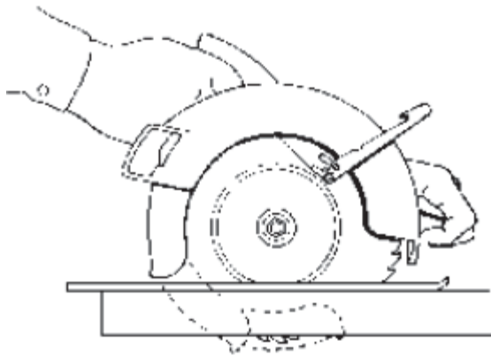
Gambar 2.7 Pelindung mesin
