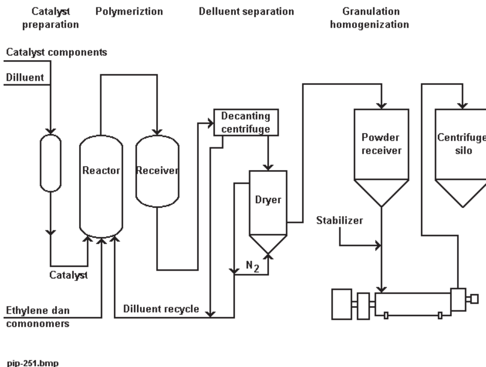
Gambar 16.14 Skema Hoechst HDPE Plant
