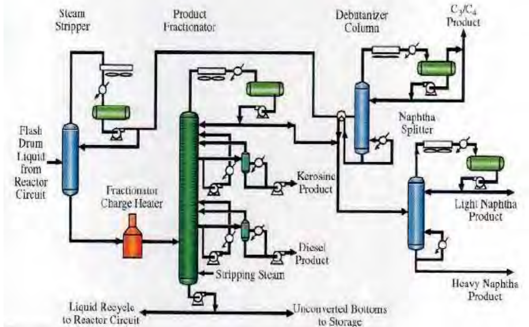
Gambar : 10 – 2 Proses Hydrocracking Seksi Fraksinasi
