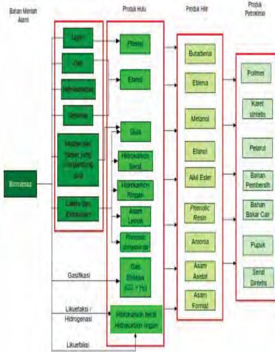
Gambar 16.6 Pohon Industri Petrokimia Berbasis Biomassa
