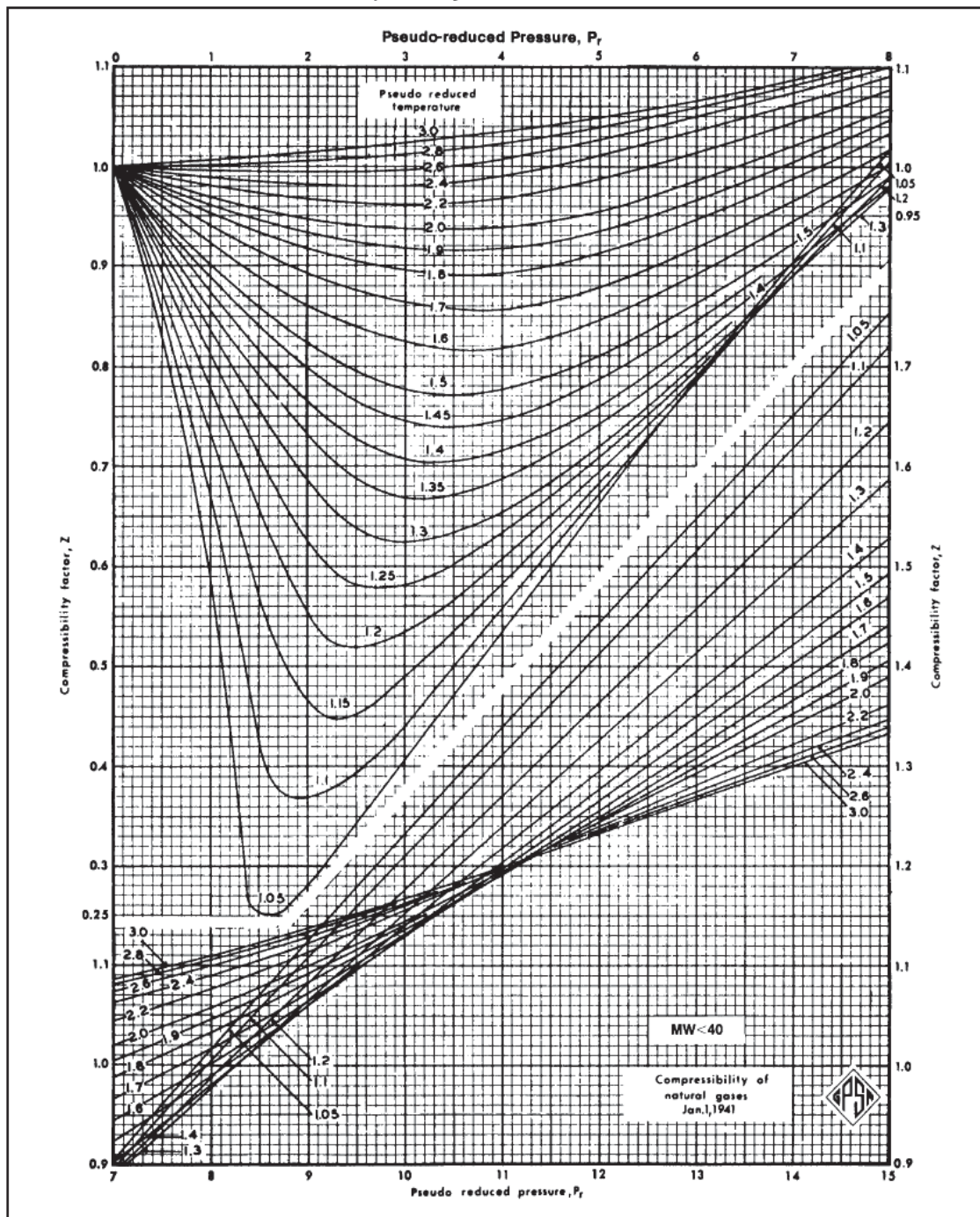
Gambar : 1 - 5 Faktor Kompresibilitas Sweet Gas
