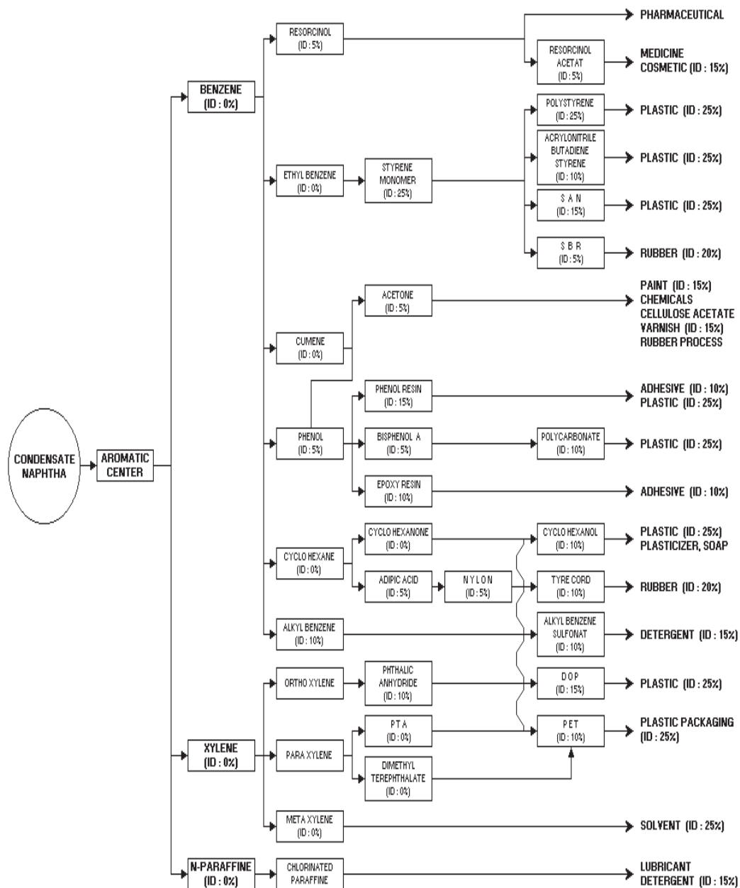
Gambar 16.5 Pohon Industri Petrokimia Hilir Aromatik
