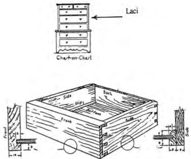
Gambar. Konstruksi Laci dan Pemasangannya
