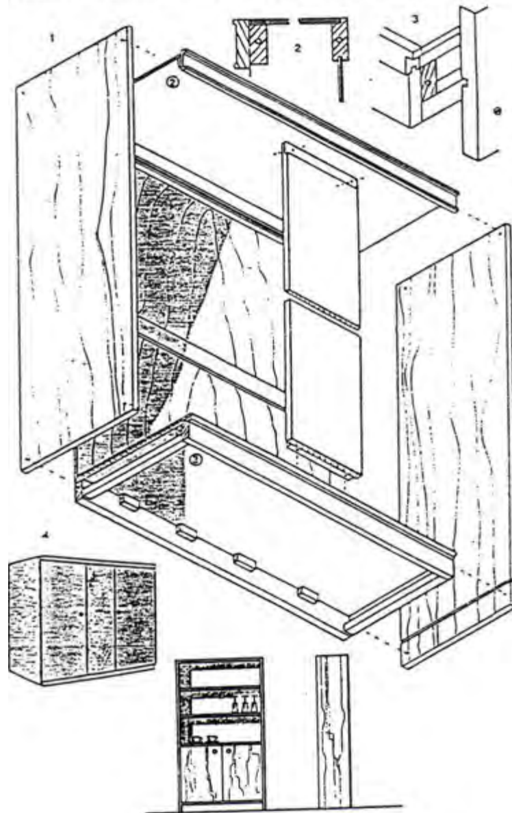
Gambar. Konstruksi Solid Carcase
