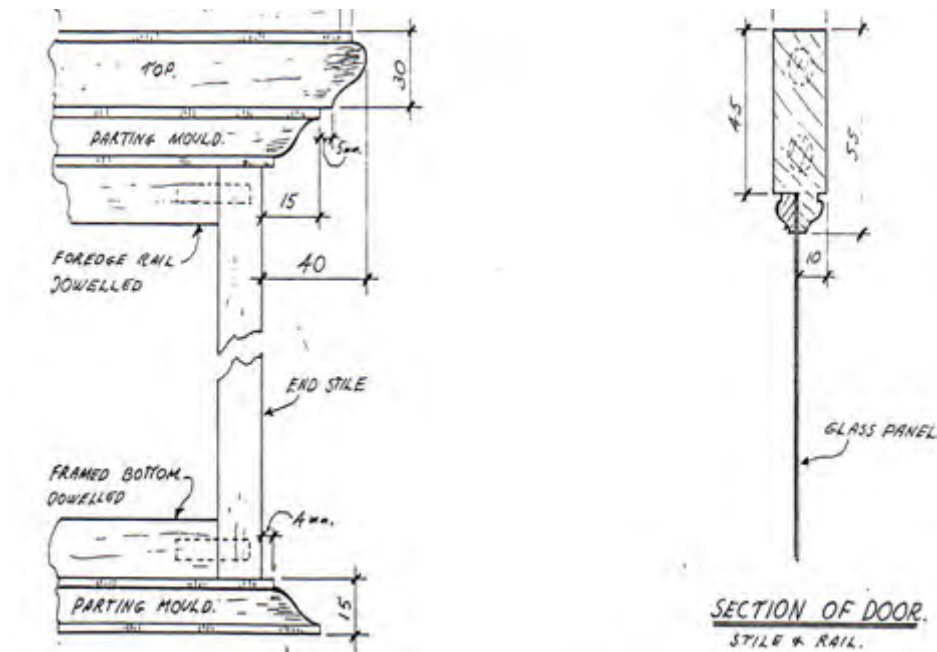
Gambar Detail Konstruksi Carcase
