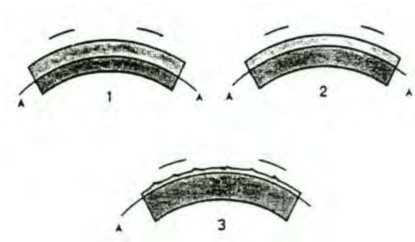
Gambar 13. Posisi Garis Netral dalam Pelengkungan kayu.
